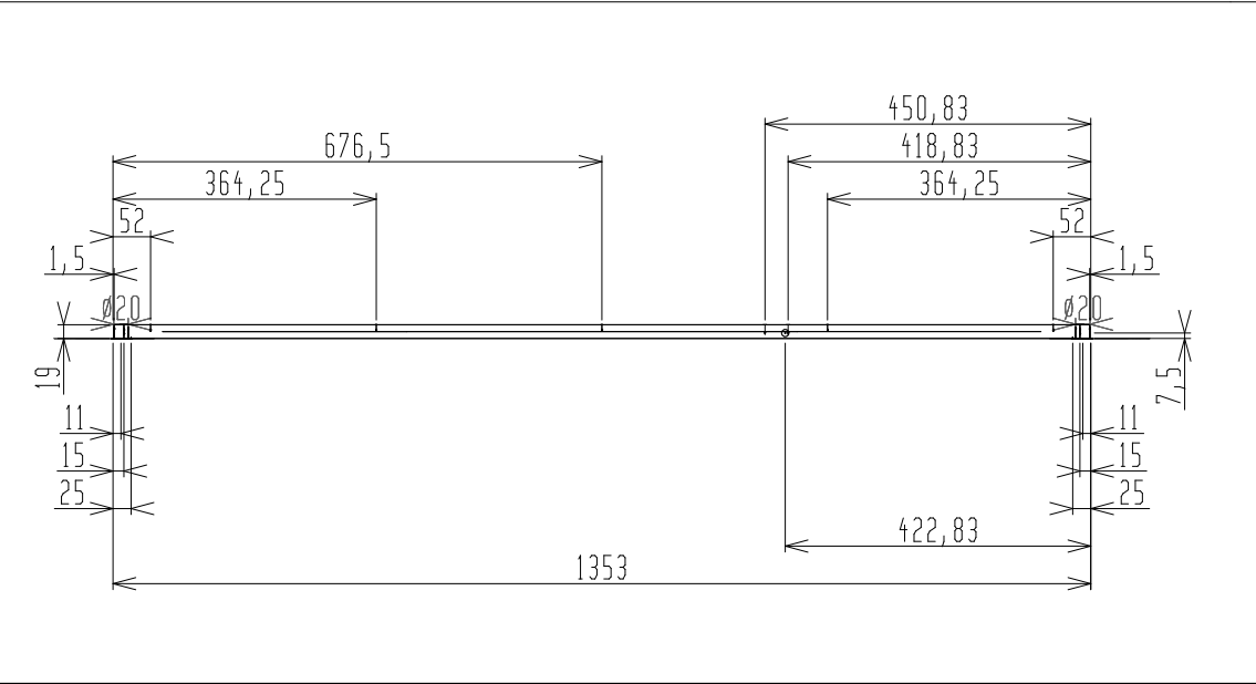
TB->Voor
