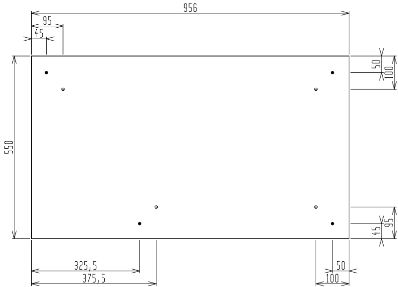
Plint->Voor
