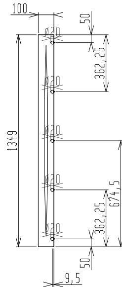
Traver_02->Voor
