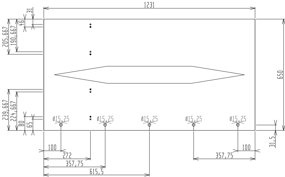
RG02->Voor
