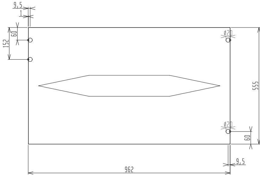
VL01->Voor
