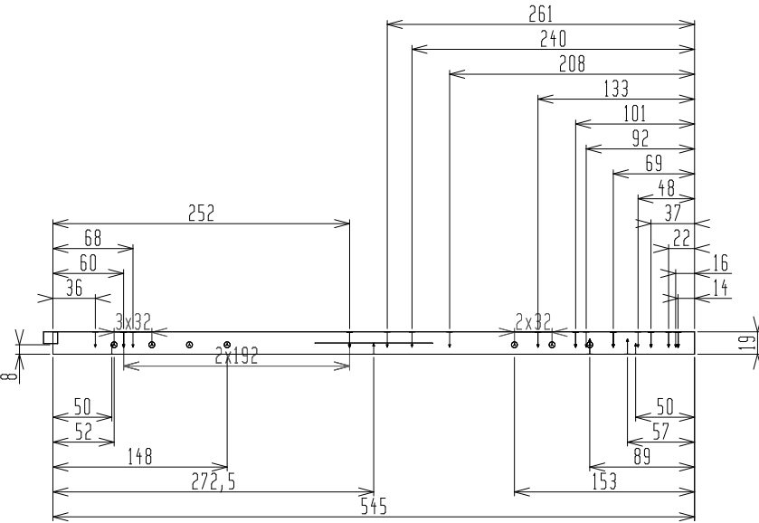
LZ->ISO
