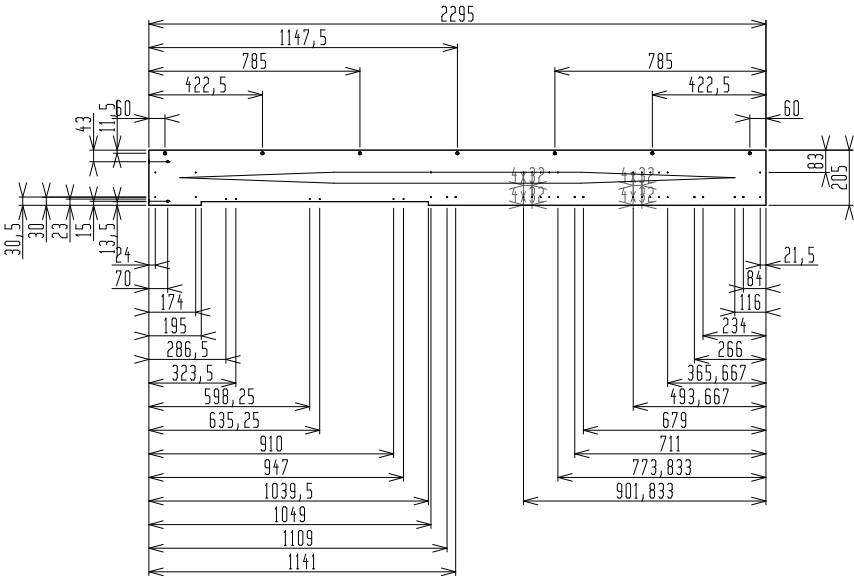
RZ->Voor
