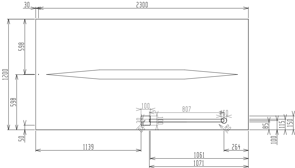
Wandplaat_02->Voor
