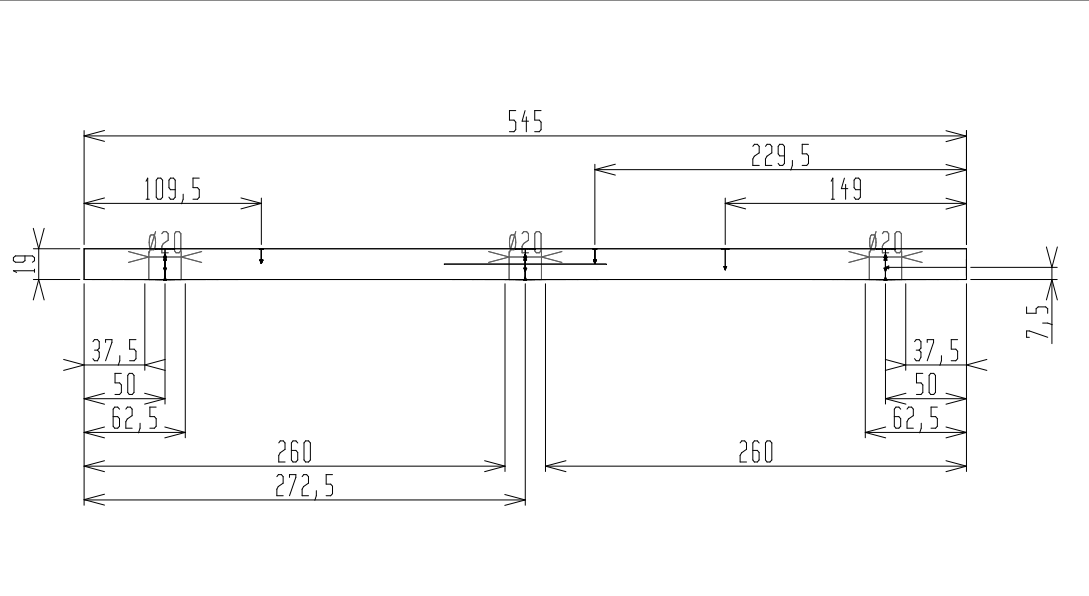
TB->ISO
