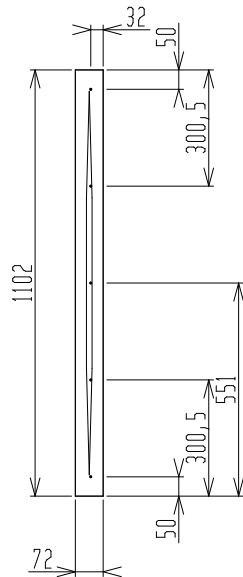
Piklat Muur->Voor
