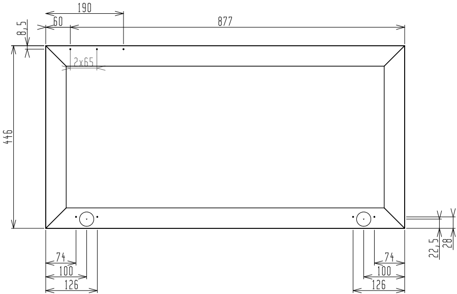
GD_R02->Voor
