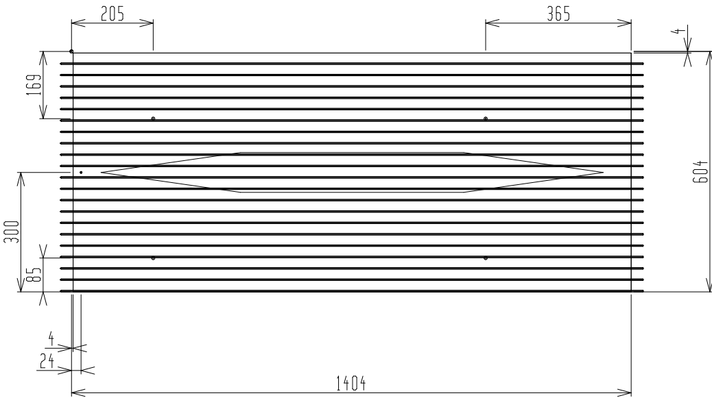
Japandi_01->Voor
