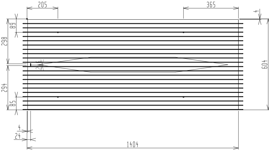
Japandi_03->Voor
