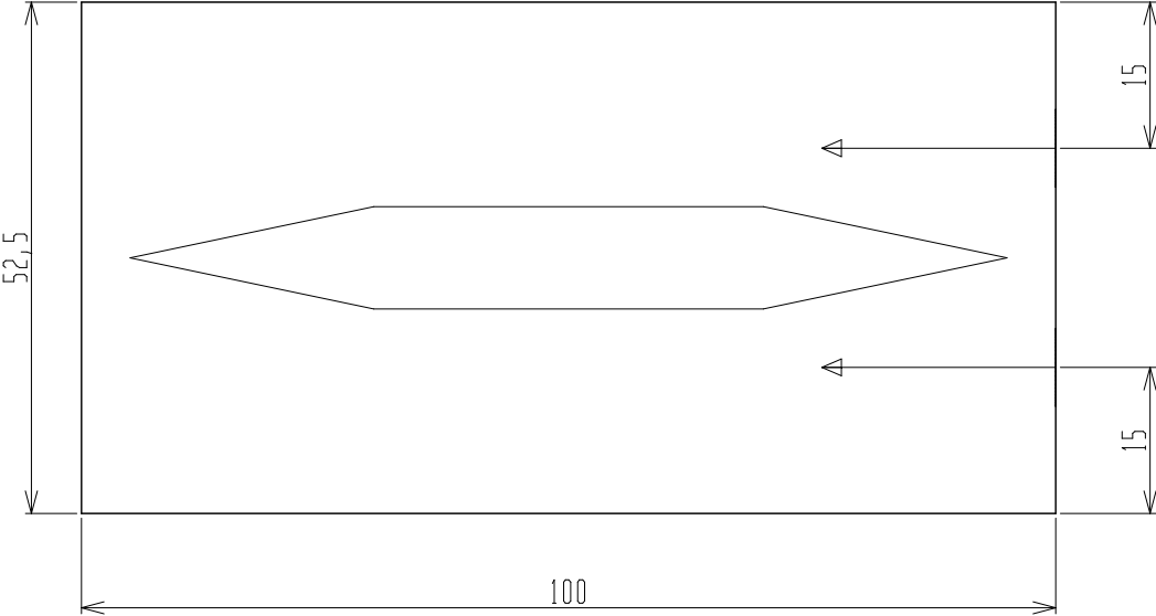
Steuntraver_02->Voor
